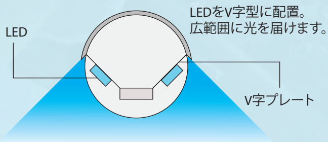
断面図
